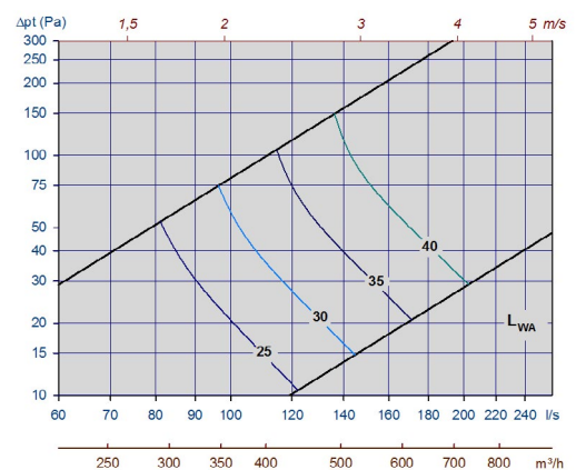
Diagram 14, Tellus-Opus-250-mid.spalthöjd
