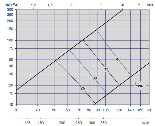
Diagram 10, Tellus-Opus-200-min.spalthöjd
