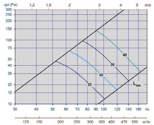
Diagram 12, Tellus-Opus-200-max.spalthöjd
